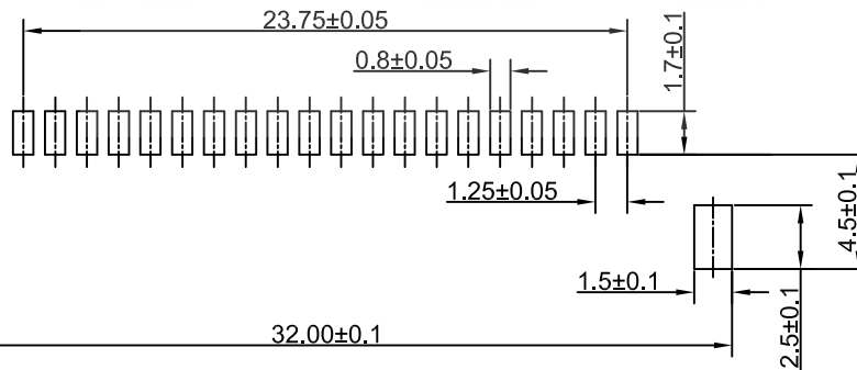
P.C.B. Dimensions layout
