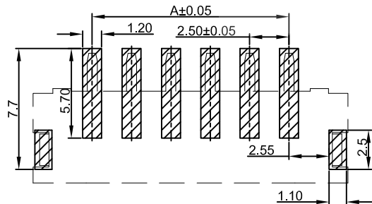
P.C.Board Layout
